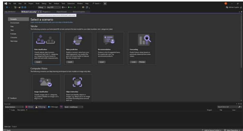
Рисунок 1 – Сценарії ML.NET
