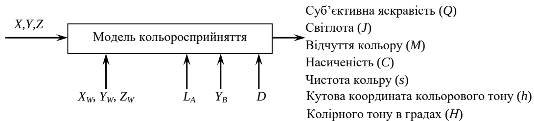
Рисунок 1.1 – Вхідні та вихідні параметри моделі кольоросприйняття CIECAM02
