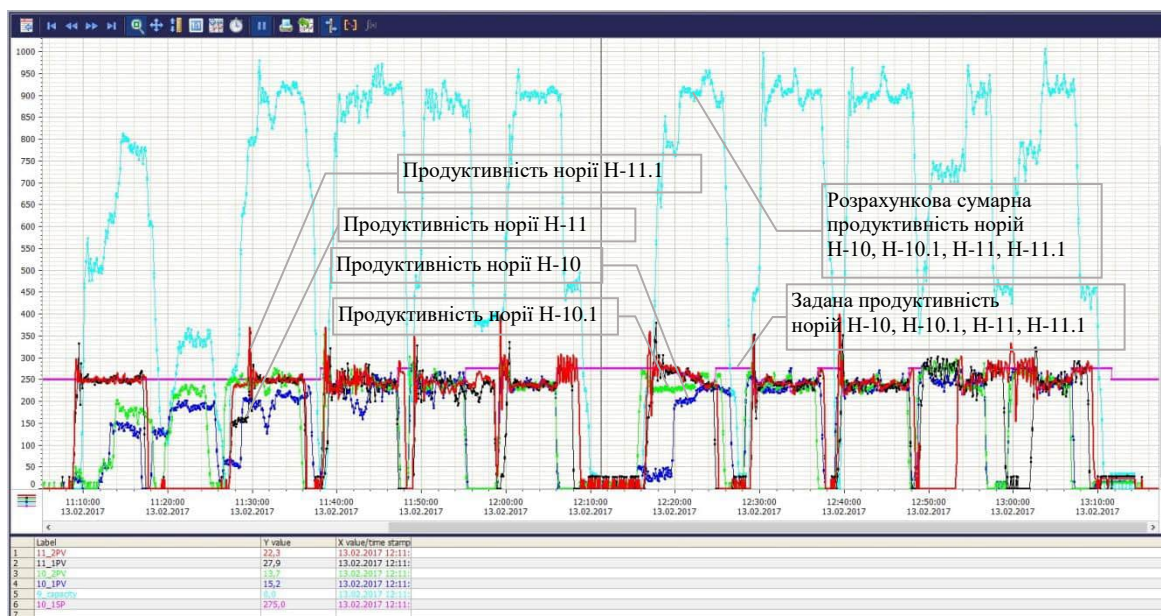
Рис. 2. Вікно «Тренди» з діаграмами зміни продуктивності норій ПТЛ перевантаження зерна із залізничного транспорту на судно при вивантаженні однієї зчіпки вагонів кукурудзи.
