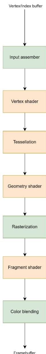
Рисунок 1 – Етапи графічного конвеєру
