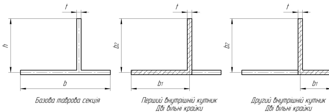
Рис. 2. Метод розбиття перерізу тавра на кутники відповідно методу Флабеля
