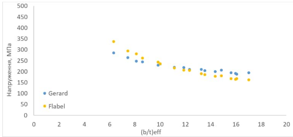
Рис. 4. Криві кріплення для профілю «ПР-113»
