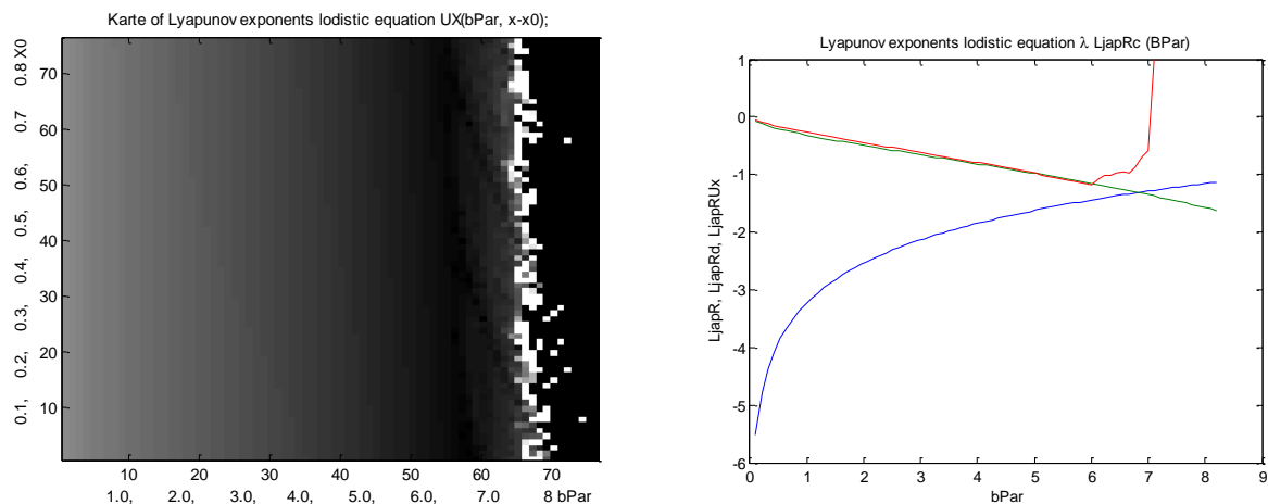
Рис. 2. Карта режимів 4-фазної системи від параметра bPar та від величини початкових значень змінних системи (ліворуч) та залежність показника Ляпунова від bPar ( max\_bPar = 8.2 ) при max\_X0 = 0.8 за величиною вхідного потоку при Xin = 0.5 (праворуч)
