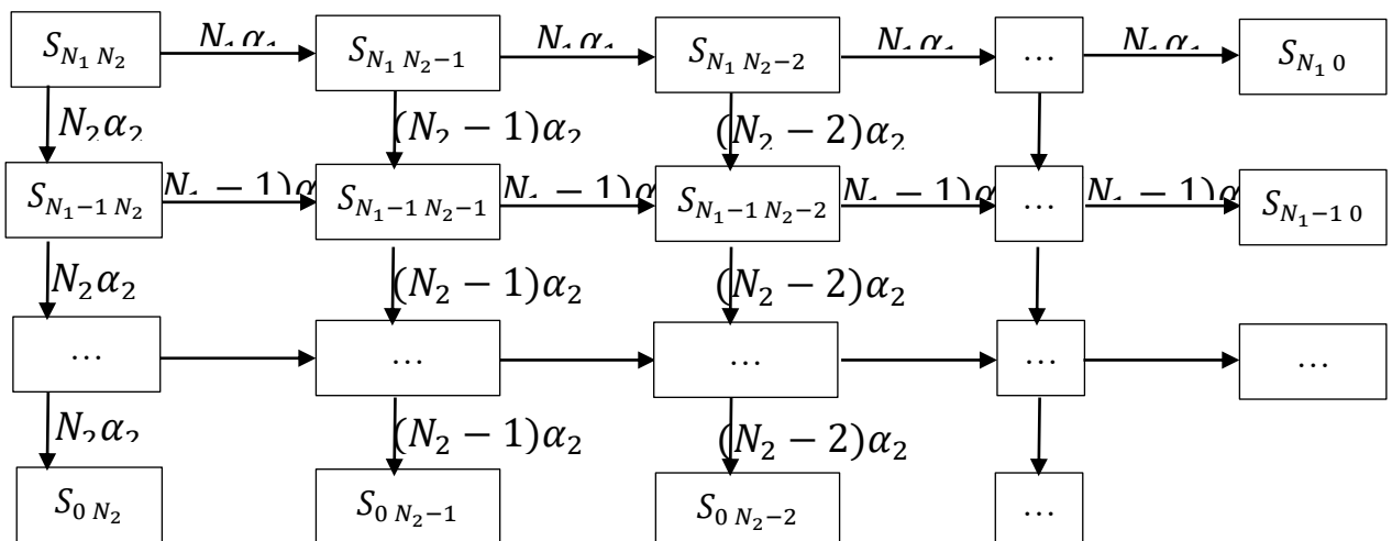
Рис. 1. – Граф станів системи, що описує бій.
