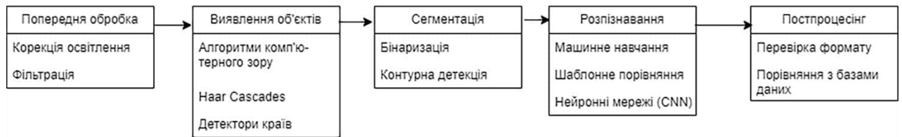
Рисунок 1 – Послідовність дій та відповідні методи для задачі розпізнавання номерних знаків
